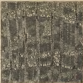
Fig. 6. - Aalaga de Europa ( Ulex europaeus , Linn.) Sección transversal. Aumento 30 diámetros.
